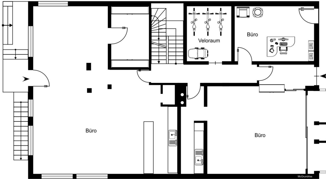
Grundriss Erdgeschoss
